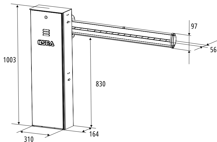
AFMETINGEN (mm)
