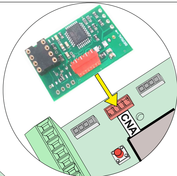
ELEKTRONISCHE STEUERUNG-BEISPIEL
